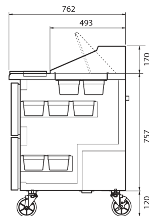
ВИД СБОКУ
