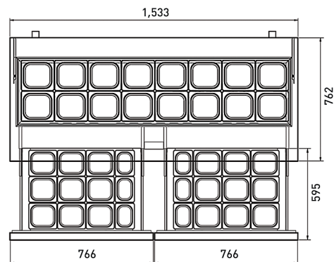
ВИД СВЕРХУ
